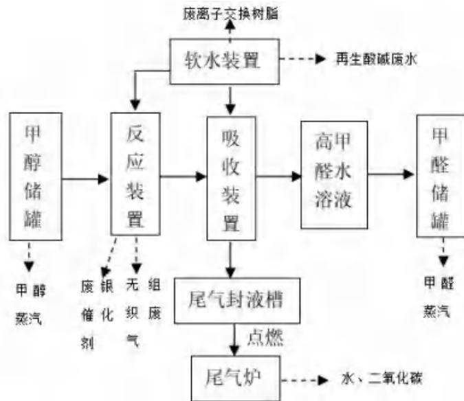
图 4.3-1 甲醛工艺流程及产污环节图
